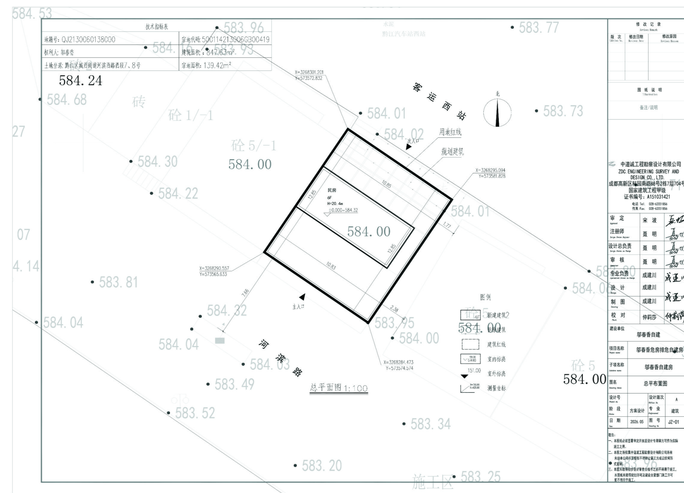
总平面图
