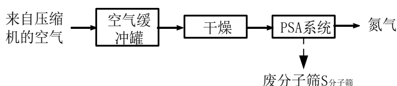
图 3.2.2-2 氮气系统工艺流程及产污环节图
