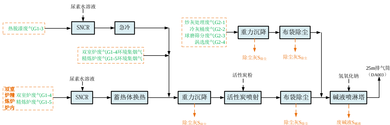
图 3.3.1-3 3#废气处理系统工艺流程简图
