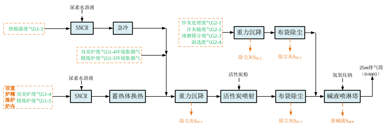
图 8.1.1-3 3#废气处理系统工艺流程简图
