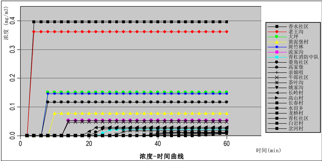
图 6.6.4.3-1 最不利气象条件下二次铝灰受潮产生氨气对敏感点的影响 mg/m 3
