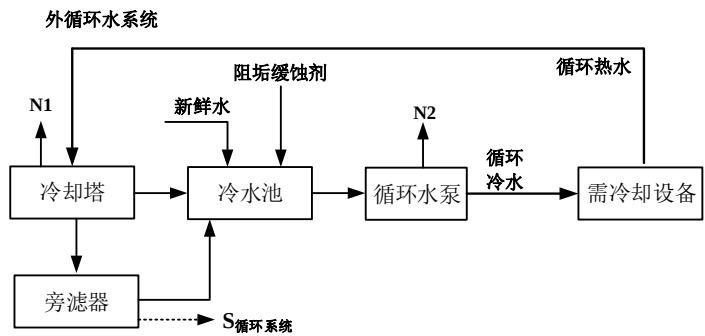
图 3.2.1-1 循环水站工艺流程及产污环节图
