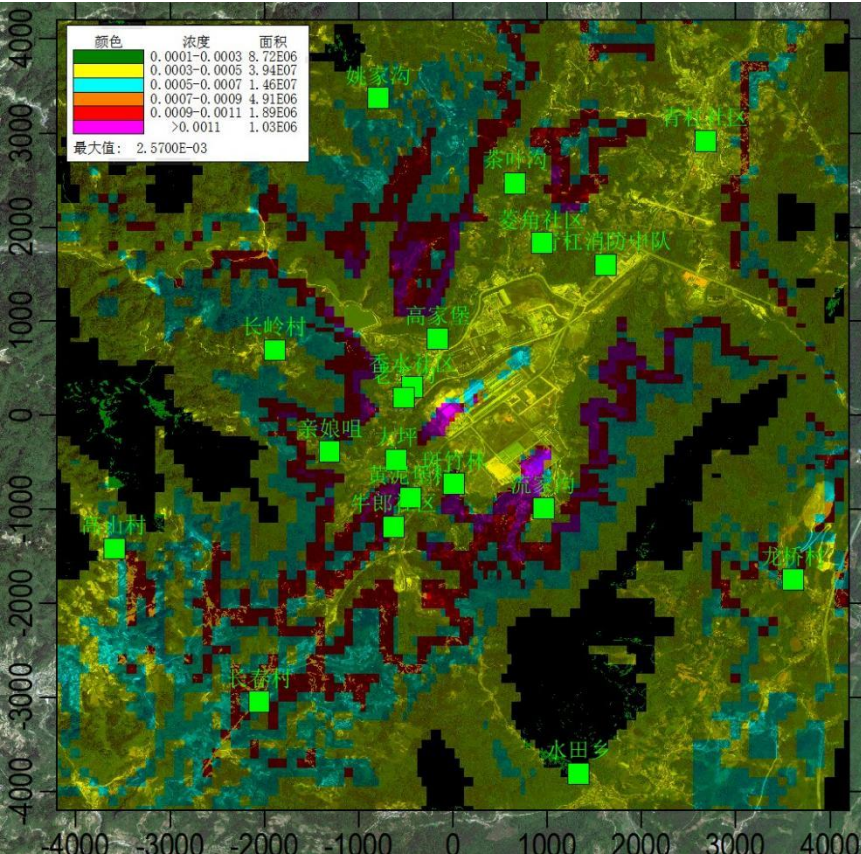
图 6.1.7-7 氟化物小时值叠加浓度网格浓度分布图
